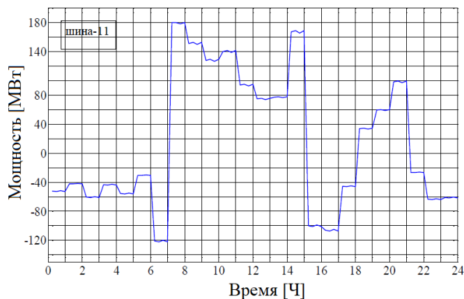
Рис.9. Изменение мощности SmartПарк на шине 11. Fig. 9. Change of SmartPark power on bus 11.
