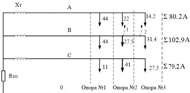
Рис.6. Симметрирование нагрузки.
