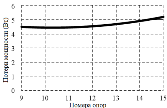
Рис.5. Потери мощности при наличии несимметричной нагрузки на разных опорах ЛЭП Fig. 5. Power losses due to asymmetric load on different power transmission poles
