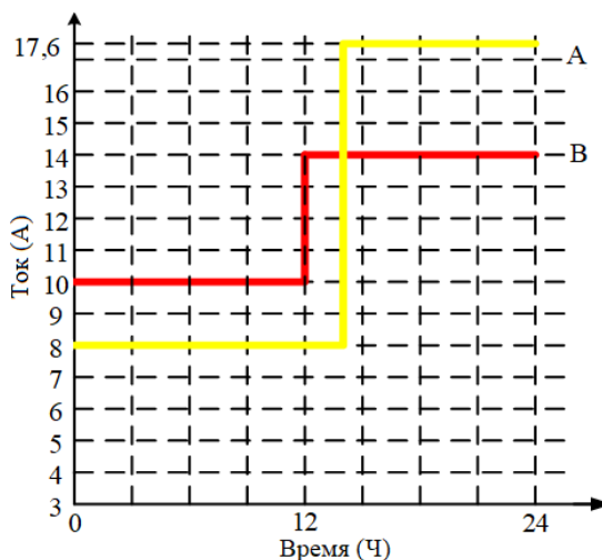
Рис.3. Нагрузки фаза А и В при разной степени загрузки в разное время. Fig.3. Load phases A and B at different loads at different times.
