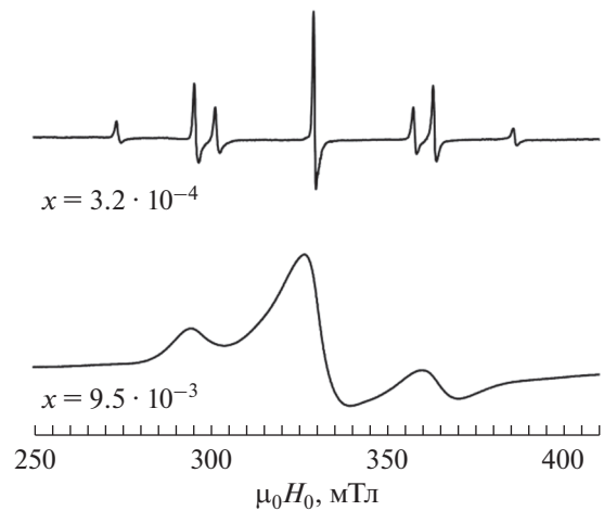
Рис. 1. Спектры ЭПР образцов № 1 и № 3 ( T = 4.2 К; H_0 \parallel \langle 001 \rangle ; f_1 = 9336 \pm 5 МГц; f_3 = 9328 \pm 5 МГц).
