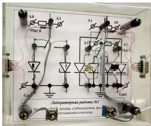
Рис. 1. Лабораторный стенд по изучению вольтамперных характеристик диодов, стабилизаторов, фотодиодов, светодиодов и оптопар
